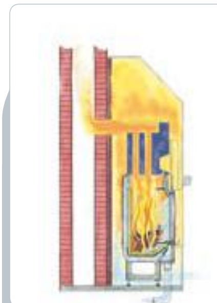
Camino con caldaia
