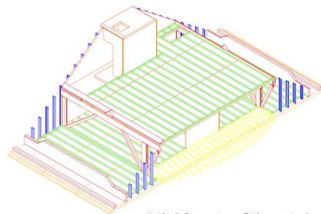
B - Vista livello mansarda pannelli X-lam e nervature ligne
